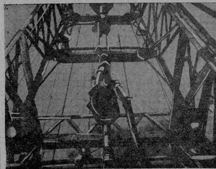
La potente grúa que estaba ayer colocando tuberías en la parte del pozo ya perforado en Chinajá, Guatemala. Trabajadores guatemaltecos dirigidos por ingenieros norteamericanos
